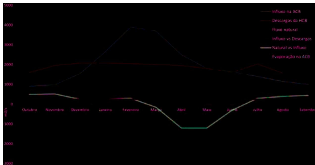
Figura 8. Fluxos médios mensais no Rio Zambeze
